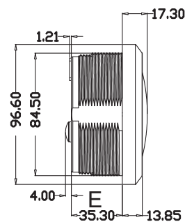
如图E:关于外形尺寸的标注说明 Picture E:Size and annotations
